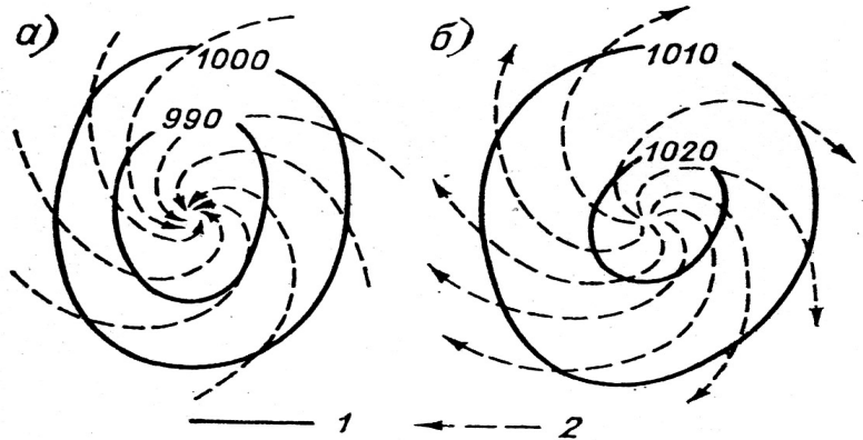
Мал. 6.18. Ізобари (1) та траєкторії перенесення повітря (2) в приземних шарах циклону (а) та антициклону (б).
