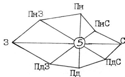
Мал. 6.10. Напрямок вітру в румбах та градусах.
