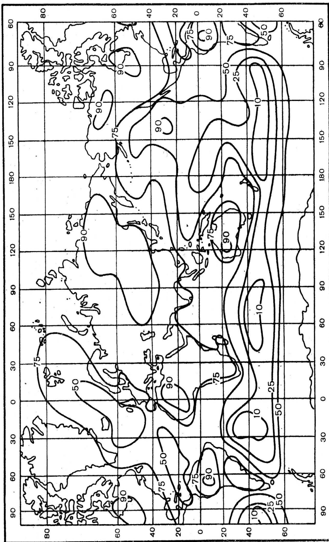
Мал.7.1.1. Континентальність клімату земної кулі за С.П. Хромовим
