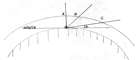
Мал. 3.3. Шлях сонячного променя в атмосфері за різної висоти Сонця над обрієм
