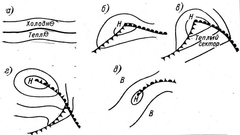
Мал. 6.33. Схема розвитку фронтальних циклонів а, б) – стадії хвилі, в) – молодий циклон, г, д) – стадії оклюзії.
