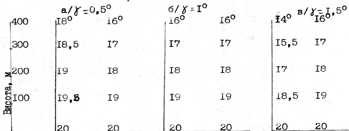
Мал. 4.11. Приклади стійкої (а), байдужої (б) та нестійкої (в) стратифікації атмосфери для ненасиченого повітря.
