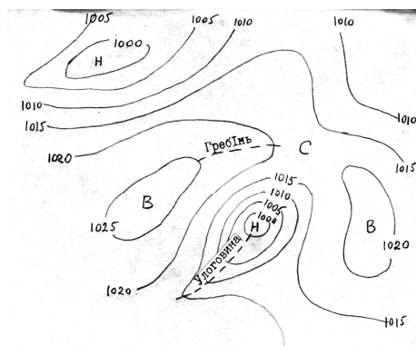
Мал. 6.2. Баричні системи на синоптичній карті: Н - циклон, В – антициклон, С – сідловина.
