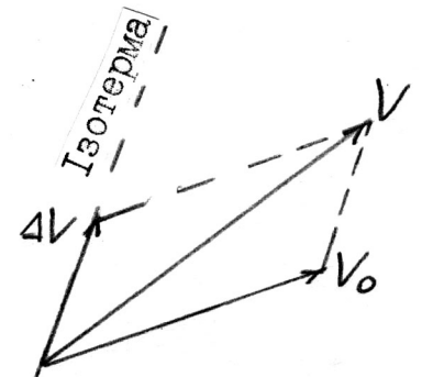
Мал. 6.15. Термічний вітер
