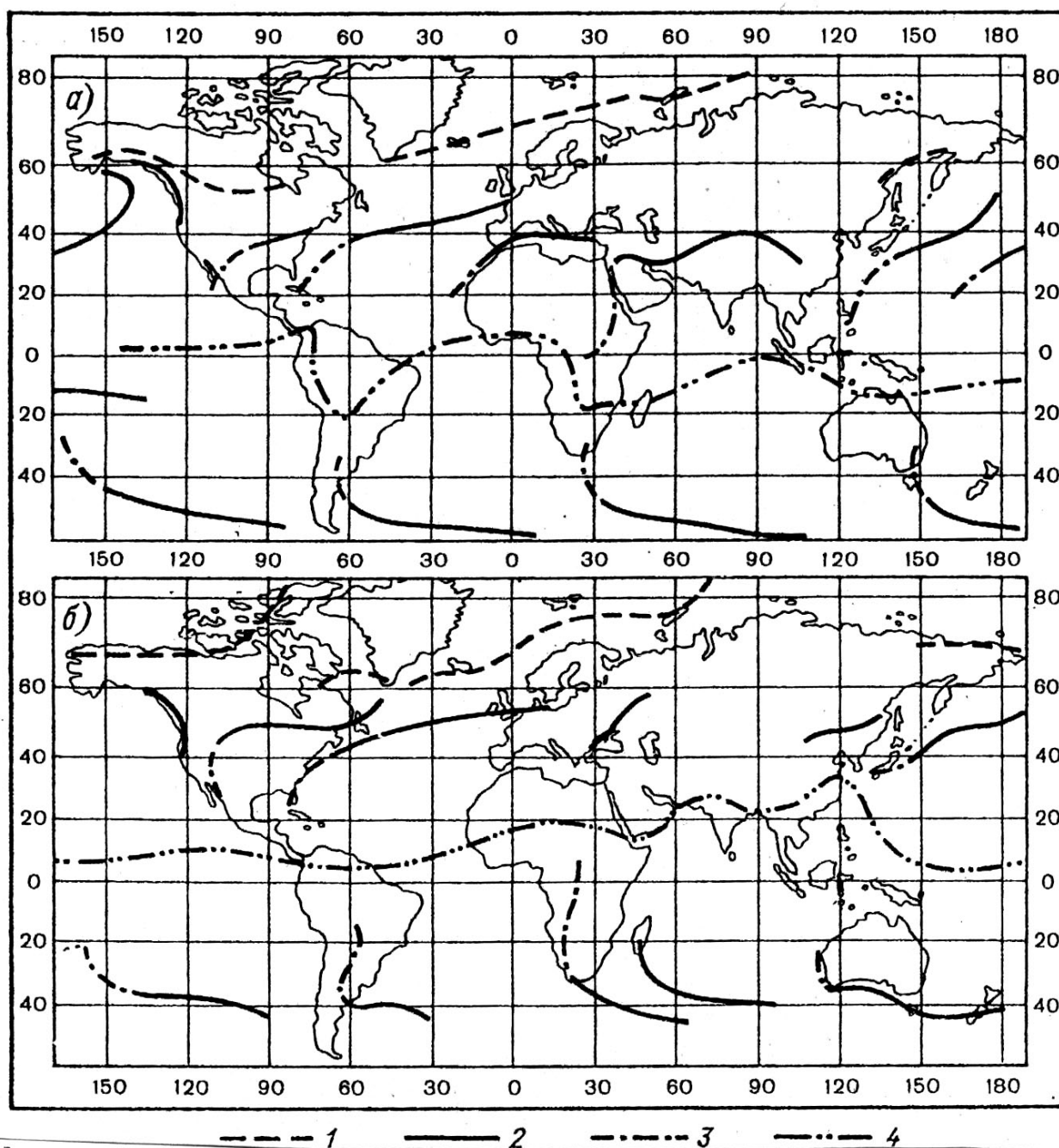
Мал. 6.25. Кліматологічні фронти: а) – січень, б) – липень. 1 – арктичний, 2 – полярний, 3 – пасатний (продовження полярного фронту в зону тропіків), 4 – тропічний.
