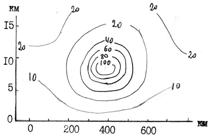
Мал. 6.22. Поперечний перетин струминної течії, м/с
