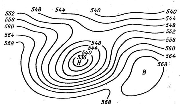
Мал. 6.4. Циклон (Н) та антициклон (В) на карті абсолютної топографії ізобаричної поверхні 500 гПа
