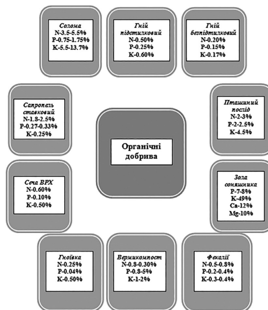
Рис. 1. Вміст NPK в органічних добривах, %/кг
