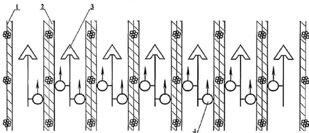
Рис. 4. Розстановка робочих органів на секції культиваторів типу КРН, КОР при наступних міжрядніх обробітках просапних культур: 1 – рядок рослин; 2 – захисна зона; 3 – універсальна стрілчаста лапа; 4 – ніж підживлювальний
