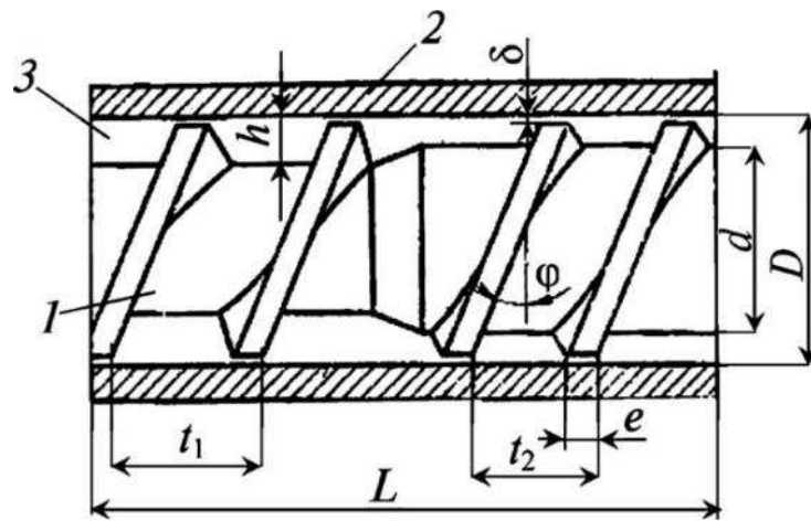
Рис. 4. Будова гвинтового каналу шнекового преса: 1 – шнек; 2 – зеєр; 3 – міжвитковий простір; h – глибина каналу; p – крок витка, що змінюється; L – довжина шнека; e – ширина витка; d – діаметр шнекового вала; D – діаметр зеєрної камери; \delta – зазор між зеєрним циліндром і витком шнека/
