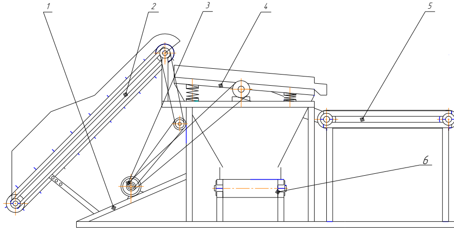
Рис. 1. – Схема однобального гiрацiйного грохота
