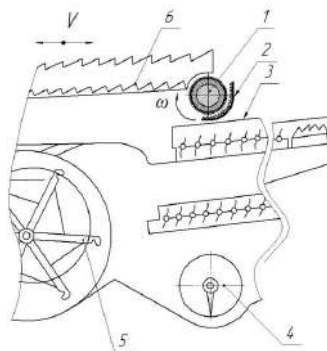
Рис. 2. Схема домолочувального пристрою люцерни в зерно-збиральному комбайні: 1 – обгумований барабан зменшеного діаметра; 2 – дека з обгумованою тірочною поверхнею; 3 – верхня решета зерноочищення; 4 – шнек; 5 – вентилятор; 6 – грохот
