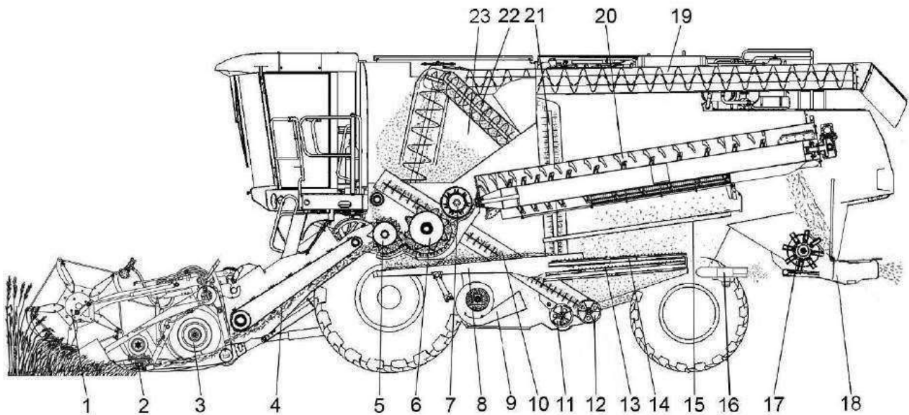
Рис. 3. Схема робочого процесу комбайна з комбінованим (гібридним) МСУ: 1 – двигун; 2 – різальний апарат; 3 – шнек; 4 – плаваючий транспортер; 5 – барабан прискорювальний; 6 – молотильний барабан; 7 – відбійний бітер; 8 – транспортна (стрясна) дошка; 9 – вентилятор; 10 – колосовий елеватор; 11 – шнек зерновий; 12 – шнек колосовий; 13 – стан решітний нижній очищення; 14 – стан решітний верхній очищення; 15 – похила дошка; 16 – полововідкидач; 17 – ротор соломорізатора; 18 – дефлектор; 19 – шнек вивантажувальний; 20 – роторні соломосепаратори; 21 – зерновий елеватор; 22 – шнек завантажувальний; 23 – бункер
