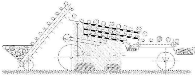
Рис. 12. Машина з робочим органом грохотного типу
