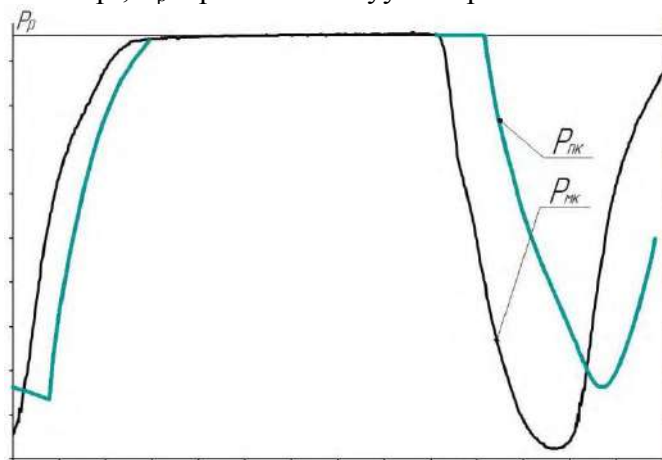
Рис. 2. Осцилограми циклічних коливань вакууму в міжстінних і підсмоктальних камерах доїльних стаканів апарату, що працює за тритактним принципом: P_{мк} – зміна вакуумметричного тиску в міжстінній камері; P_{пк} – зміна вакуумметричного тиску в підсмоктальній камері; P_p – робочий вакуумметричний тиск.
