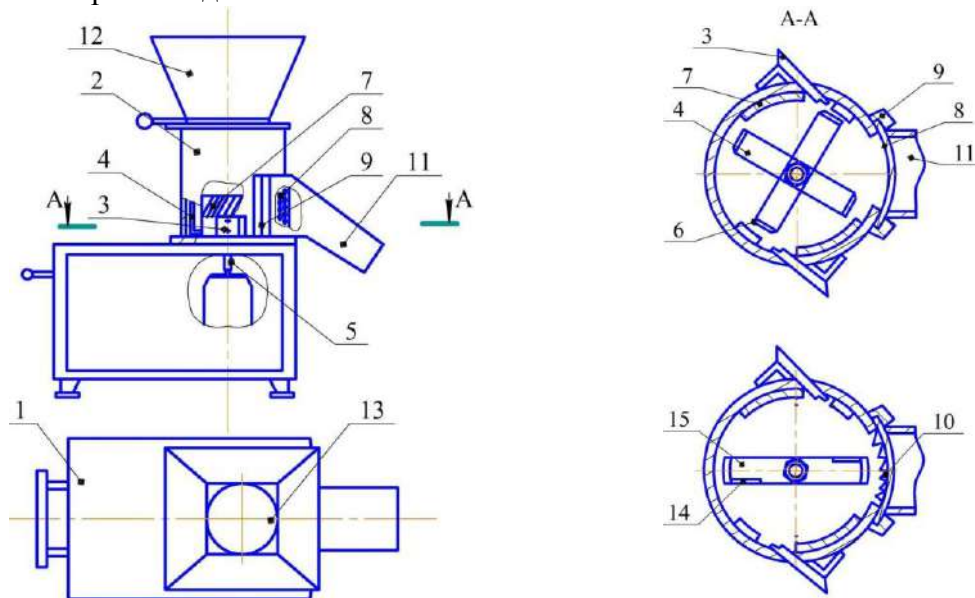
Рис. 1. Універсальний подрібнювач кормів: 1 – основа; 2 – дробильна камера; 3 – бічні ножі; 4 – хрестоподібний ніж; 5 – вал; 7 – знімні накладки; 8 – змінні решета; 9 – напрямні; 10 – шинкування; 11 – знімний рукав; 12 – знімний бункер; 13 – шибер; 14 – знімний ніж; 15 – додаткові вертикальні ребра.
