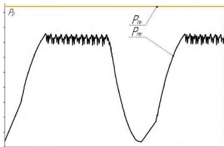
Рис. 3. Осцилограми циклічних коливань у міжстінних і підсоскових камерах доїльних стаканів апарата АДУ-1-04 (PulsoTest Comfort): P_{мк} – зміна вакуумметричного тиску в міжстінній камері; P_{пк} – зміна вакуумметричного тиску в підсосковій камері; P_p – робочий вакуумметричний тиск.
