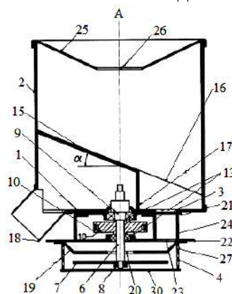
Рис. 2. Пристрій для подрібнення сільськогосподарської продукції за патентом № 2252073: 1 – станина; 2 – бункер; 3 – вікно; 4 – сито; 5 – електродвигун; 6 – вал; 7 – ударна пластина; 8 – гайка; 10, 11 – шків; 12 – ремінна передача; 13 – підшипники; 9 – отвір; 14 – посадкова площадка; 15 – знімне днище; 16 – виріз; 17 – перегородка; 18 – лоток; 19 – мембрана; 20 – отвір; 21 – заслінка; 22 – пластина; 23 – вікно для зерна; 24 – перегородка; 25 – кришка; 26 – отвір для засипання зерна; 27 – отвори перфорації; 28 – шпилька; 29 – шнур; 30 – дно; 31 – захисний козирок.
