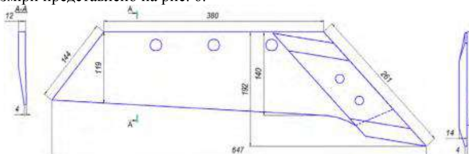
Рис. 6. Леміш фірми "Vogel i Noot"
