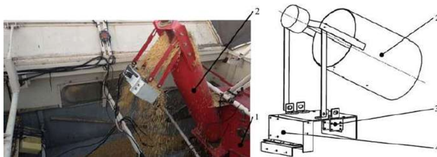
Рис. 1. Вид та структурна схема проовідбірника зерна
