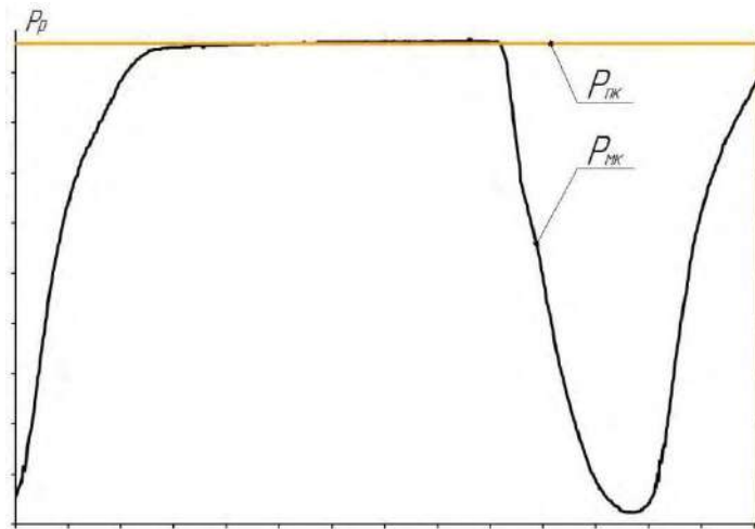
Рис. 1. Осцилограми циклічних коливань вакууму в міжстінних і підсискових камерах доїльних стаканів апарату, що працює за двотактним принципом (PulsoTest Comfort): P_{мк} – зміна вакуумметричного тиску в міжстінній камері; P_{пк} – зміна вакуумметричного тиску в підсисковій камері; P_p – робочий вакуумметричний тиск.
