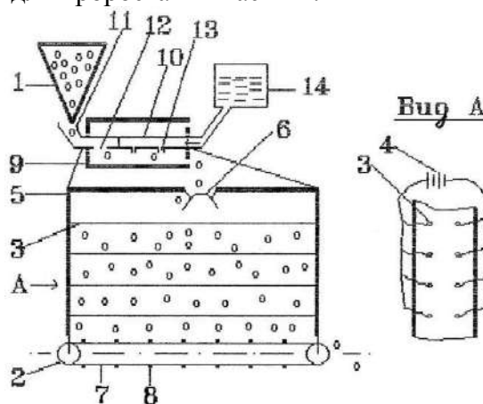
Рис. 6. Пристрій електричної обробки
