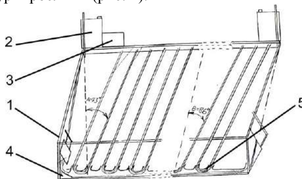
Рис. 4. Схема пристрою контактної дії для нанесення концентрованих гербіцидів: 1 – каркас; 2 – вертикальні резервуари; 3 – насос; 4 – колекторна рамка; 5 – кінцеві чашки
