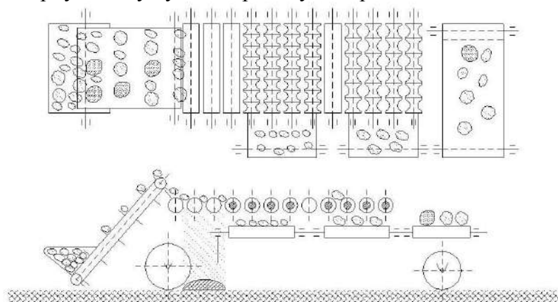
Рис. 6. Сортувальний пристрій із роликowym робочим органом
