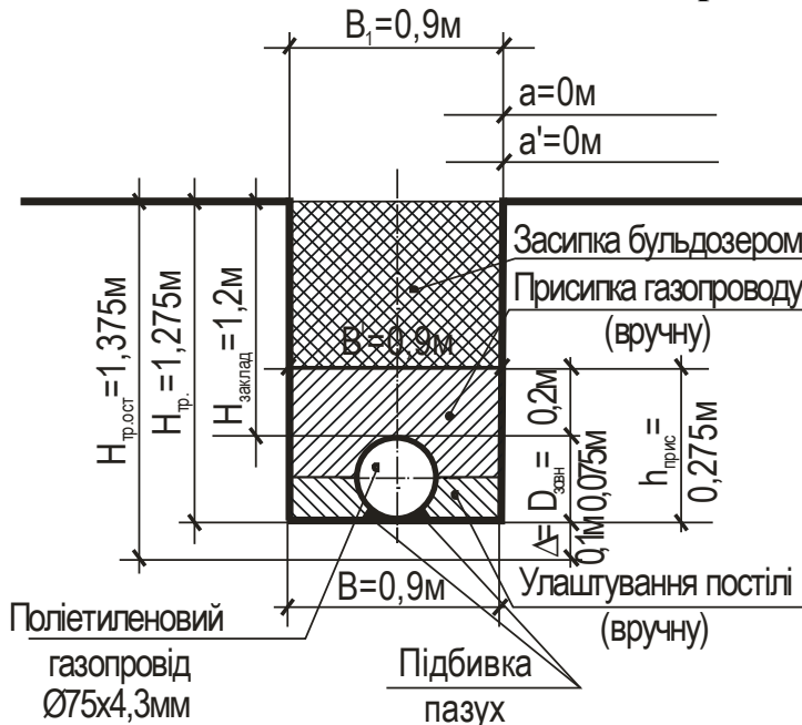
Рис. 2.1 Поперечний переріз траншеї
